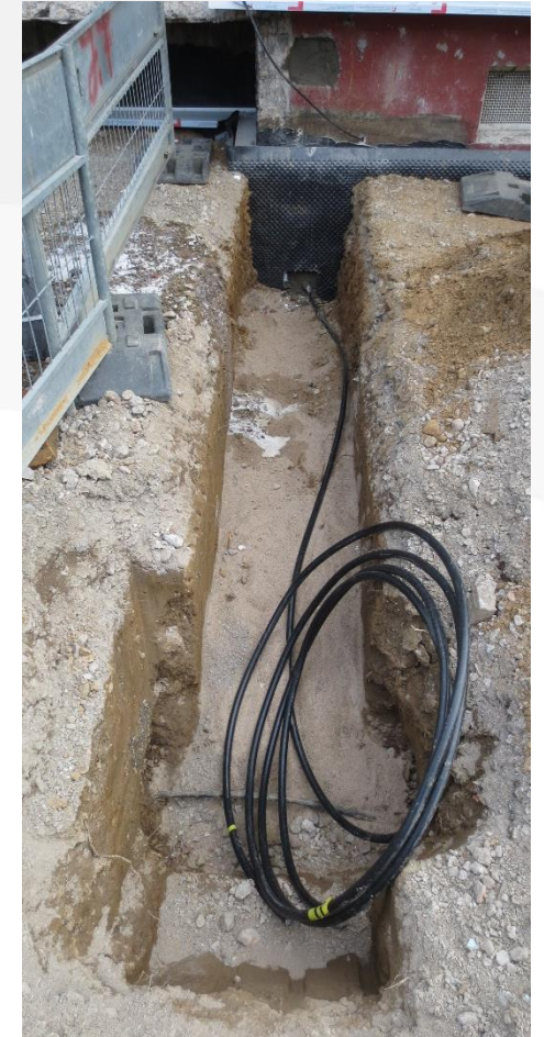
Neubau + Leerrohr
